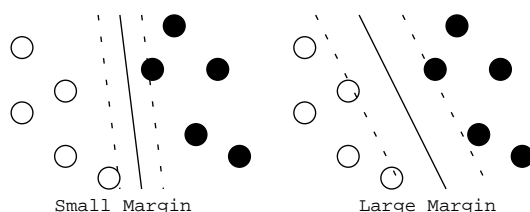
図 1 マージン最大化
